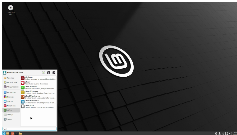
Fig. 3: Xfce
