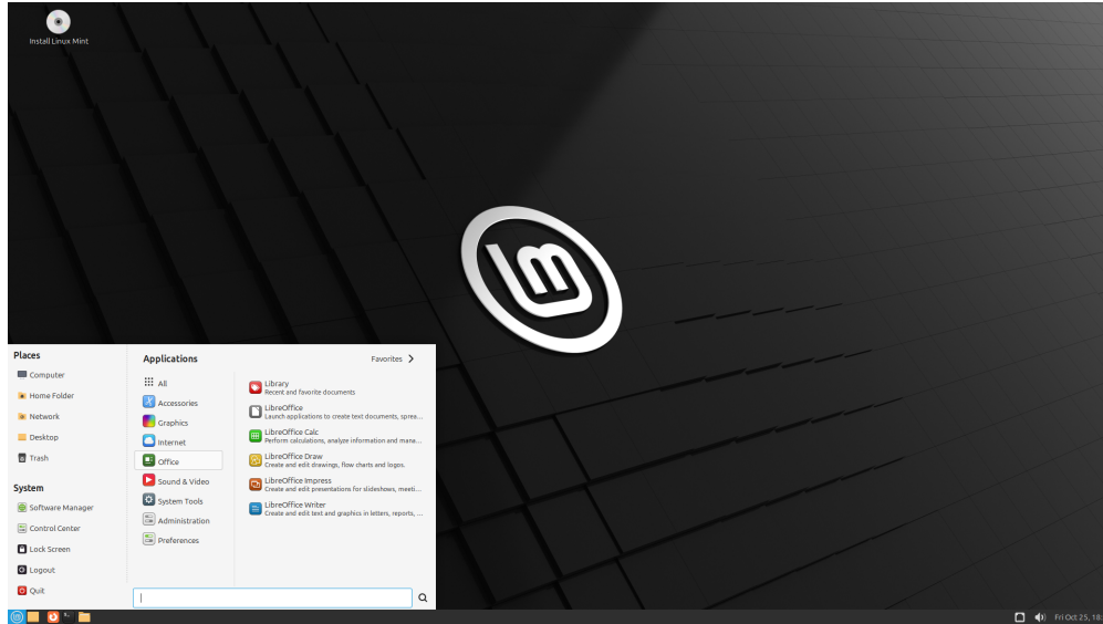
Fig. 2: MATE
